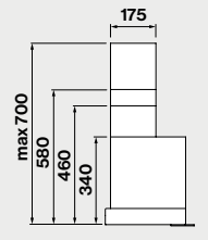
Vista laterale con camino opzionale
