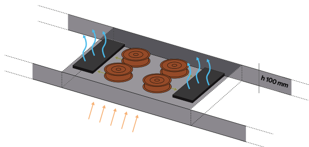
Filtrazione Multi-Air. 4 motori ultracompatti e 2 filtri Carbon.Zeo
