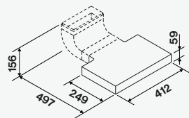
Foro per incasso griglia
