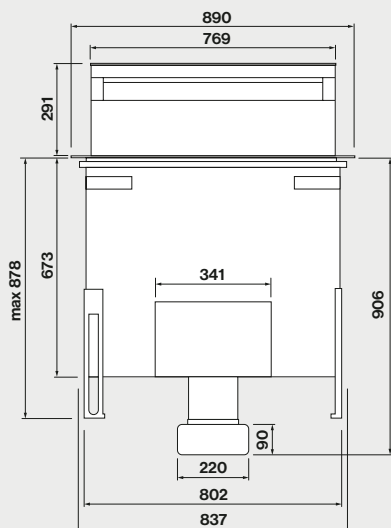
Vista laterale con motore in posizione anteriore
