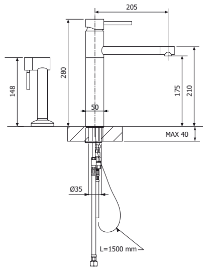
Miscelatore monocomando lavello cucina 2-fori > doccetta esterna monogetto 2-holes single lever sink mixer > one-jet side-spray
