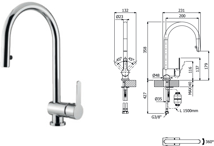
Miscelatore monocomando lavello cucina > doccetta estraibile monogetto in ABS > canna C
