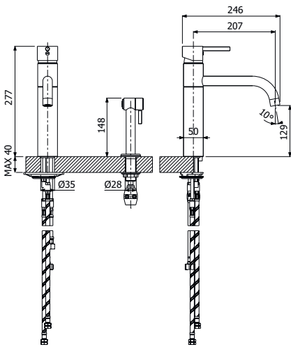
Miscelatore monocomando lavello cucina 2-fori > doccetta esterna monogetto 2-holes single lever sink mixer > one-jet side-spray
