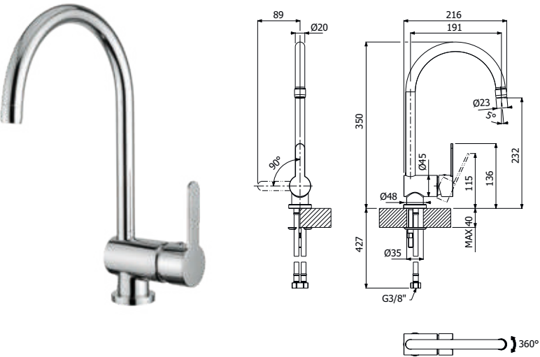
Miscelatore monocomando lavello cucina > canna C
