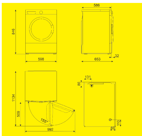
LB1T82AIT
