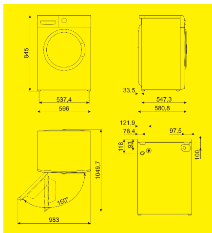
DR92EIT
