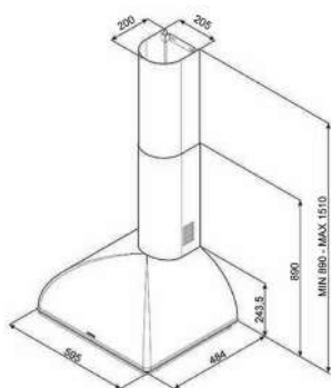
KS59
