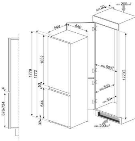
C41721E
