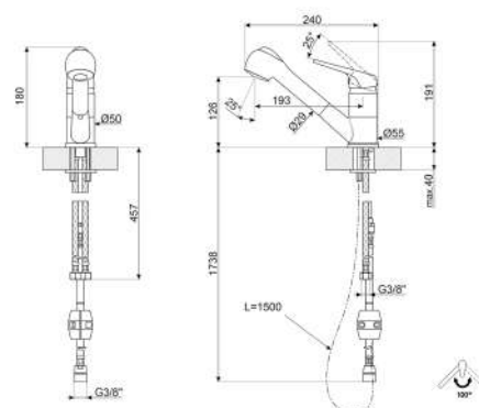
MD10
