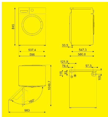
DN82SE
