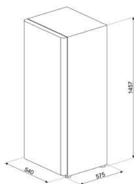
CV215NE
