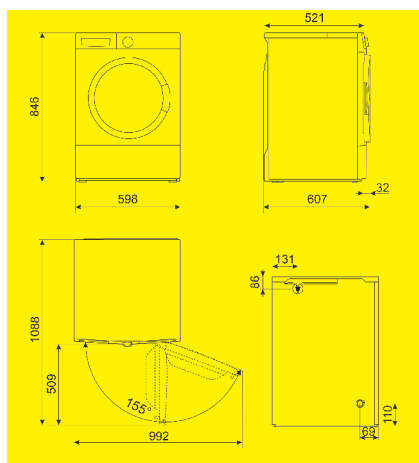
DN93SE
